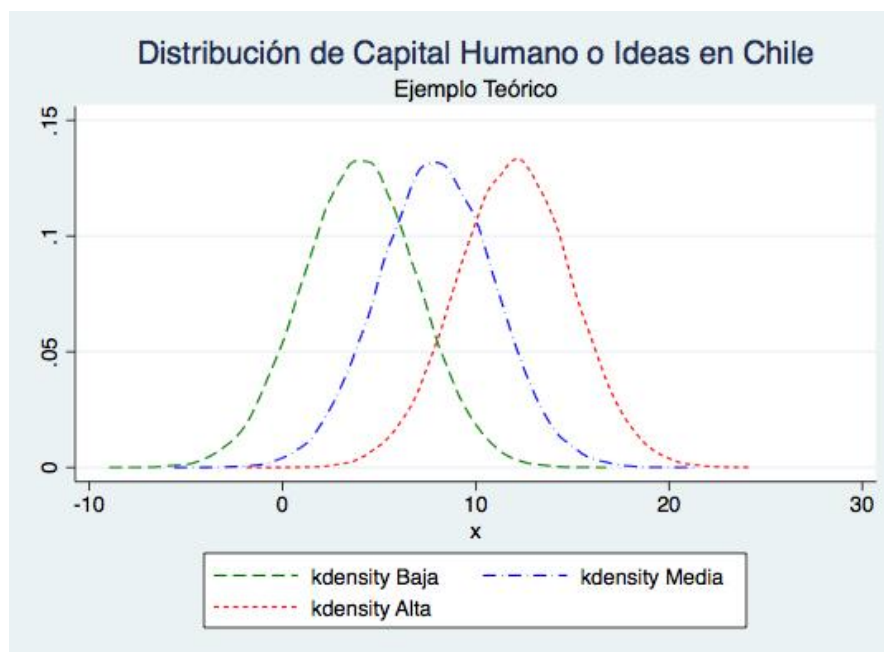
Gráfico I: Ejemplo Teórico de la Desigualdad
